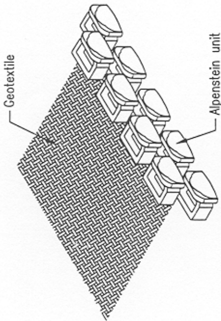
ISOMETRIC ASSEMBLY DETAIL N.T.S.
